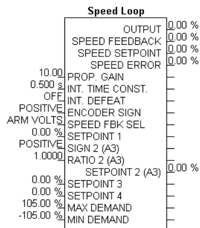
图19 速度环功能块
